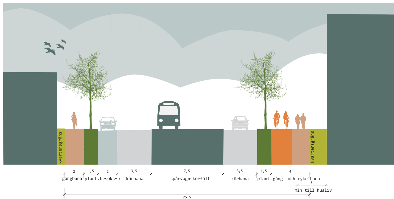
sektion Litteraturgatan söder
