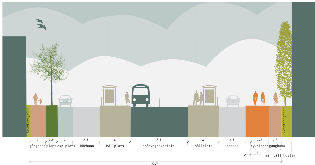
sektion Litteraturgatan hållplatsen
