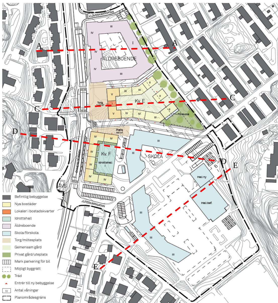
Illustrationskarta över den södra delen av planområdet med redovisning av sektioner A-A till E-E. Semrén & Månsson
