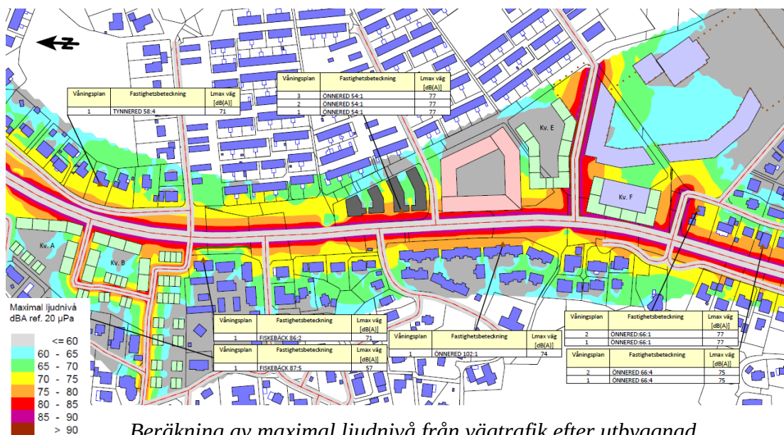
Beräkning av maximal ljudnivå från vägtrafik efter utbyggnad.
