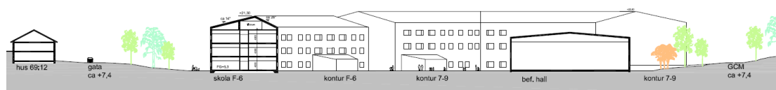
Sektion E-E genom F-6 skola och idrotts hall. Norconsult
