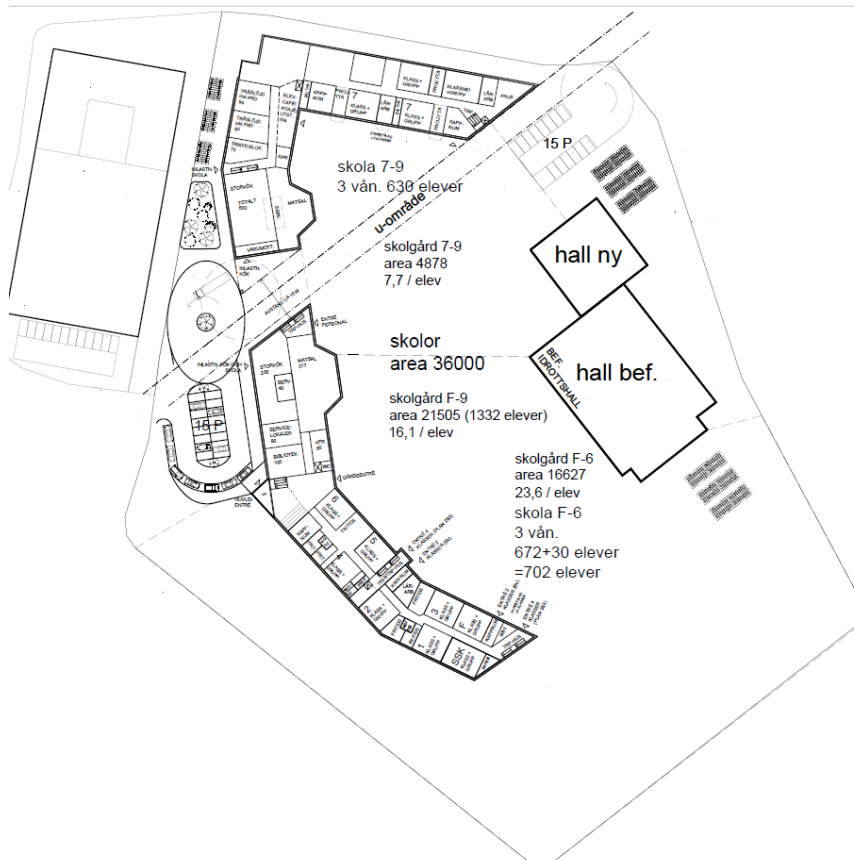
Karta över föreslagna skolbyggnader samt skolgård. Norconsult
