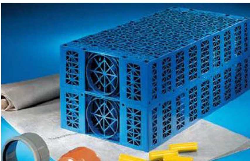
Figur 6. Dagvattenkassetter. Källa: www.wavin.se .
