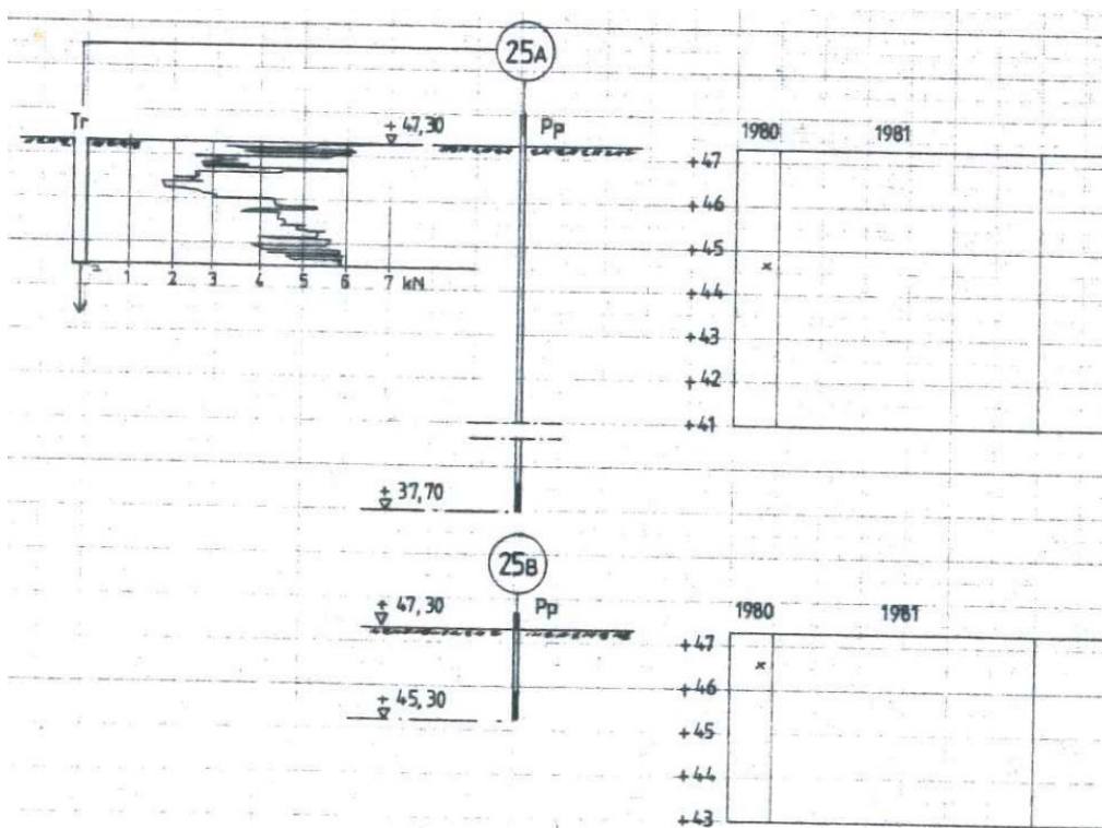
GAMMALT GW-RÖR 25
