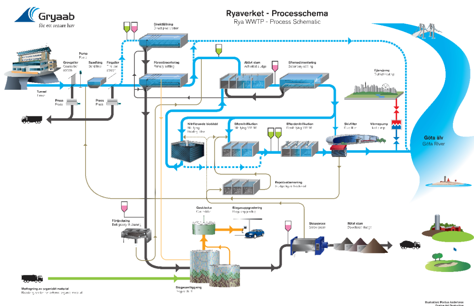
Figur 27 Processchema om flödesvägar genom Ryaverket. Tjocka blåa linjen presenterar huvudflödesvägen av vatten och bruna flödesvägar av slam. Streckade linjen presenterar möjliga vägar för förbildning av flöden.
