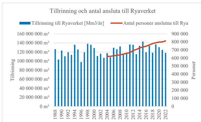
Figur 30 Tillrinning till Ryaverket sedan 1988 och ansluten befolkning.
