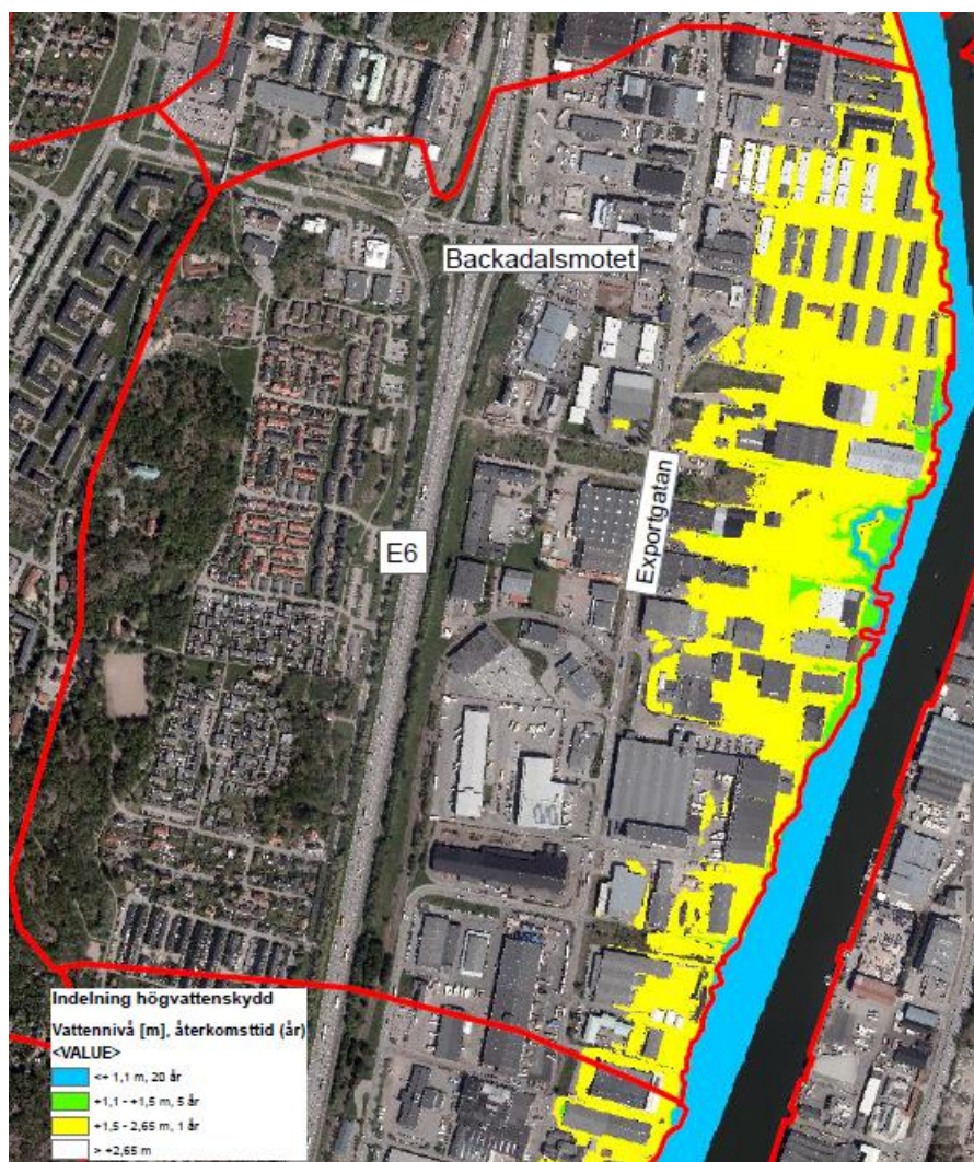
Figur 6. Indelning av högvattenskydd efter återkomsttid och vattennivå inom Exportgatans avrinningsområde år 2100.
