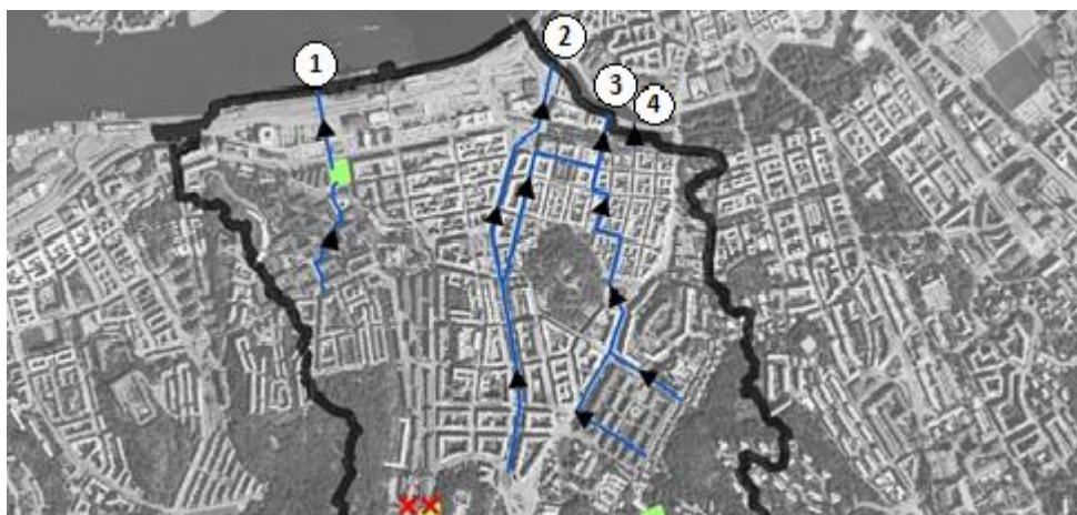
Figur 18. Nedre delen av Linnéstaden avrinningsområde. Siffror 1–4 visar skyfallsledningarnas utlopp till Göta älv och Rosenlundskanalen.
