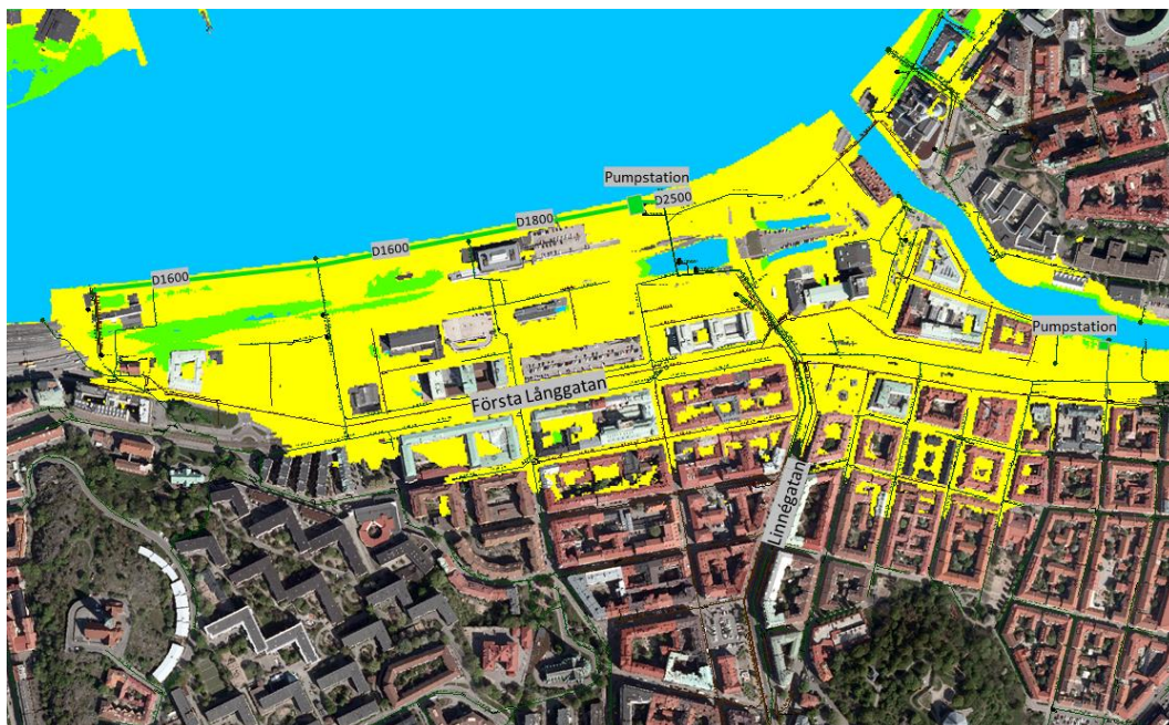
Figur 19. Principlösning för Linnéstaden avrinningsområde, med en större pumpstation för 4 stycken utlopp som samlas ihop med avskärande ledningar, samt en mindre som pumpar till Rosenlundskanalen. Ledningsdimensioner med minsta lutning på 1 ‰ för självrensning framgår av kartan.
