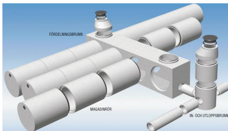
Figur 25. Exempel på utjämningsmagasin bestående av rörpaket i betong (Alfarör).
