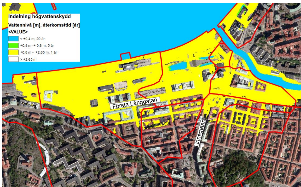
Figur 9. Indelning av högvattenskydd efter återkomsttid och vattennivå inom Linnéstadsens avrinningsområde med dagens klimat.
