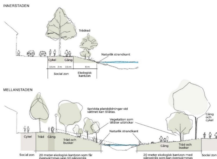
Figur 2. Principsektioner för blågröna stråk för innerstaden och mellanstaden, från Göteborgs översiktsplan. I innerstaden bör minst 13 meter kantzon på båda sidor eftersträvas varav 6 meter ekologisk kantzon. För att möjliggöra och utveckla vistelseytor längs med stråken krävs en bredare kantzon än så.
