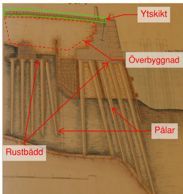
Figur 1: Principskiss kanalmur med definitioner, ur Kulturmiljö utredning Antiquum, 2021-11-22
