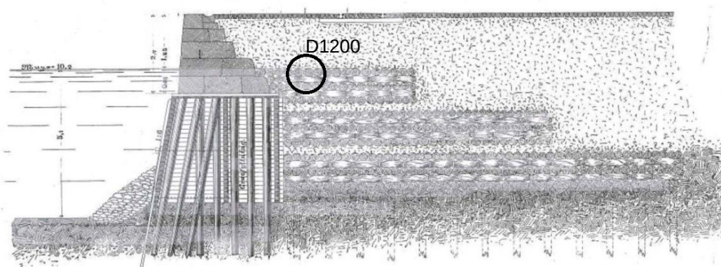
Figur 26 Placering avskärande ledning dimension 1200 med placering i Packhuskajen.
