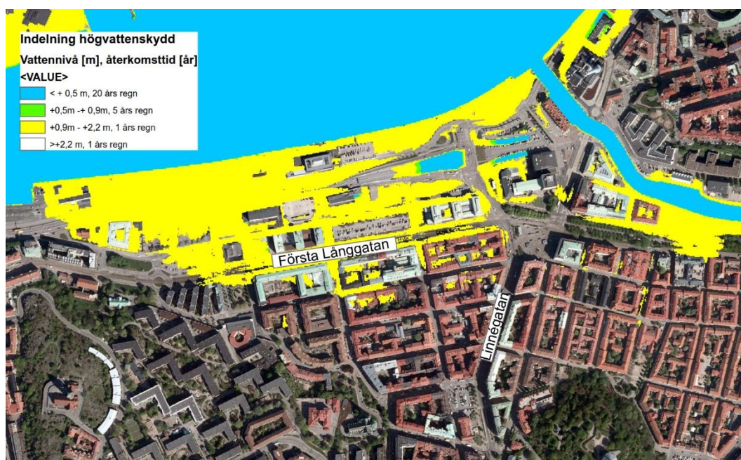
Figur 11. Indelning av högvattenskydd efter återkomsttid och vattennivå inom Linnéstadens avrinningsområde till år 2040.
