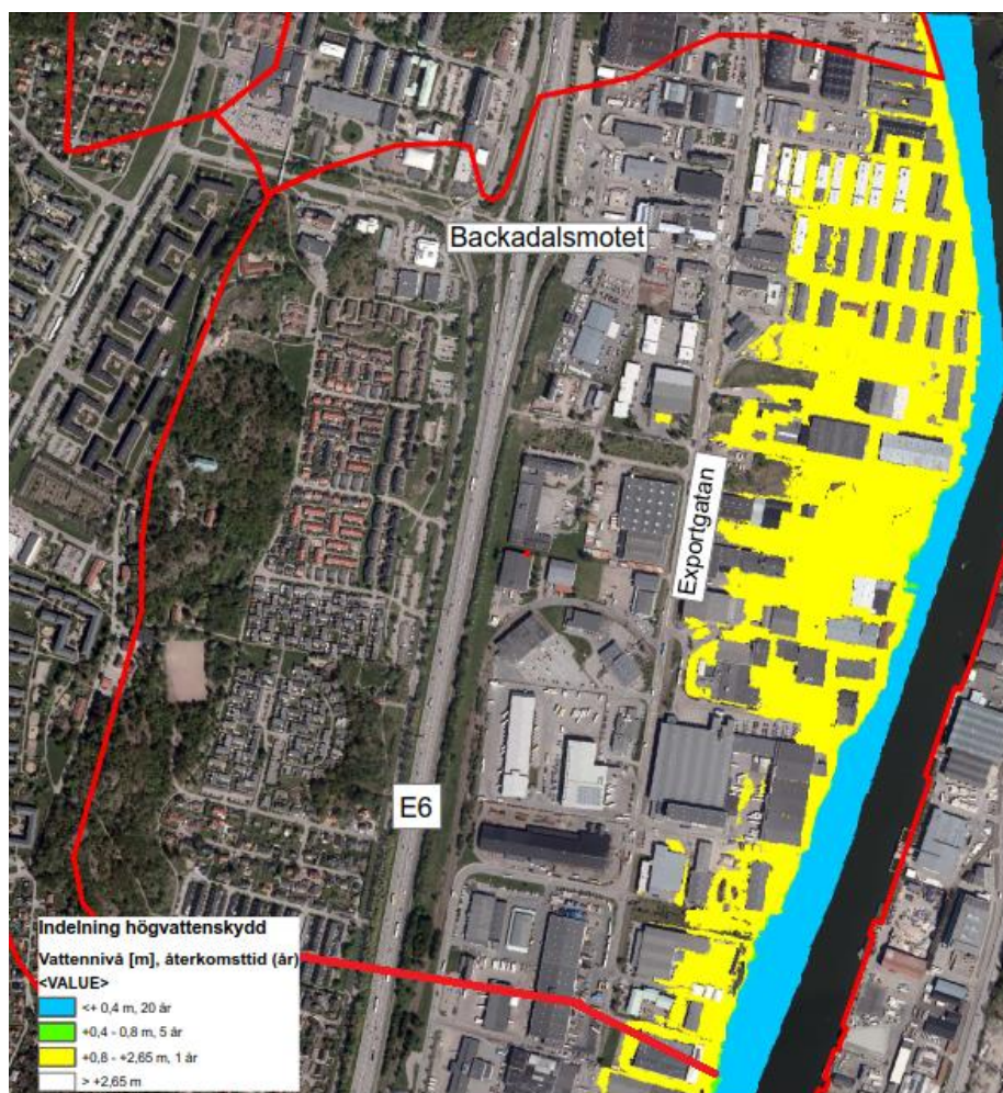
Figur 5 Indelning av högvattenskydd efter återkomsttid för regn vid olika vattennivåer inom Exportgatans avrinningsområde med dagens klimat.
