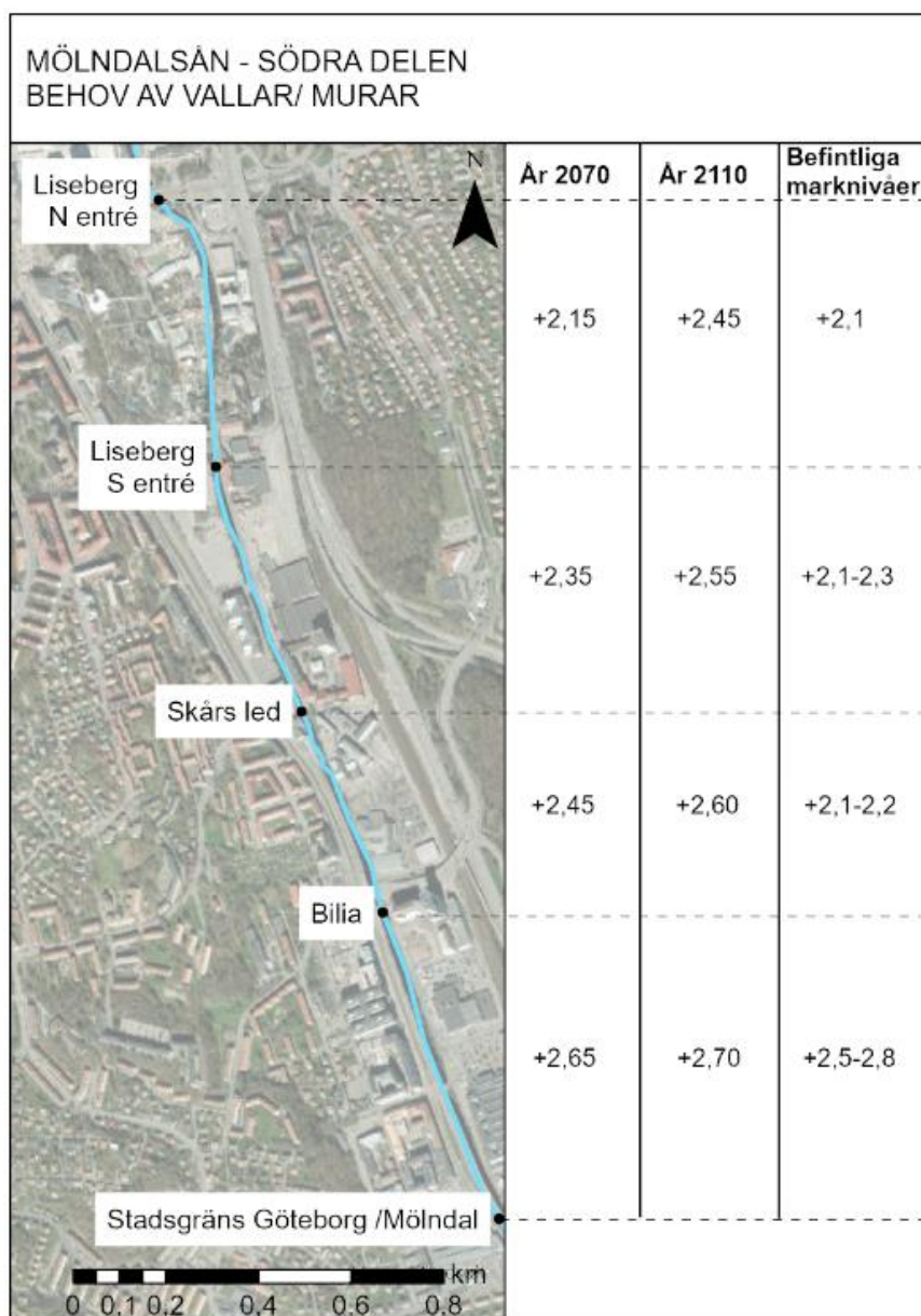
Figur 3-2. Detaljkarta över erforderliga nivåer på vallar/murar år 2070 och som ett alternativ år 2110 till följd av höga flöden (ej skyfall) om planer på pumpning skjuts på framtiden. Jämförelse med befintliga marknivåer
