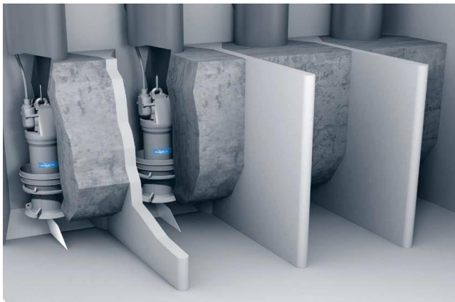
Figur 22 T.v. kolumnpumpar med inloppsbrunn i betong, t.h. lågtryckspump N 3301 (Källa: Flygt)
