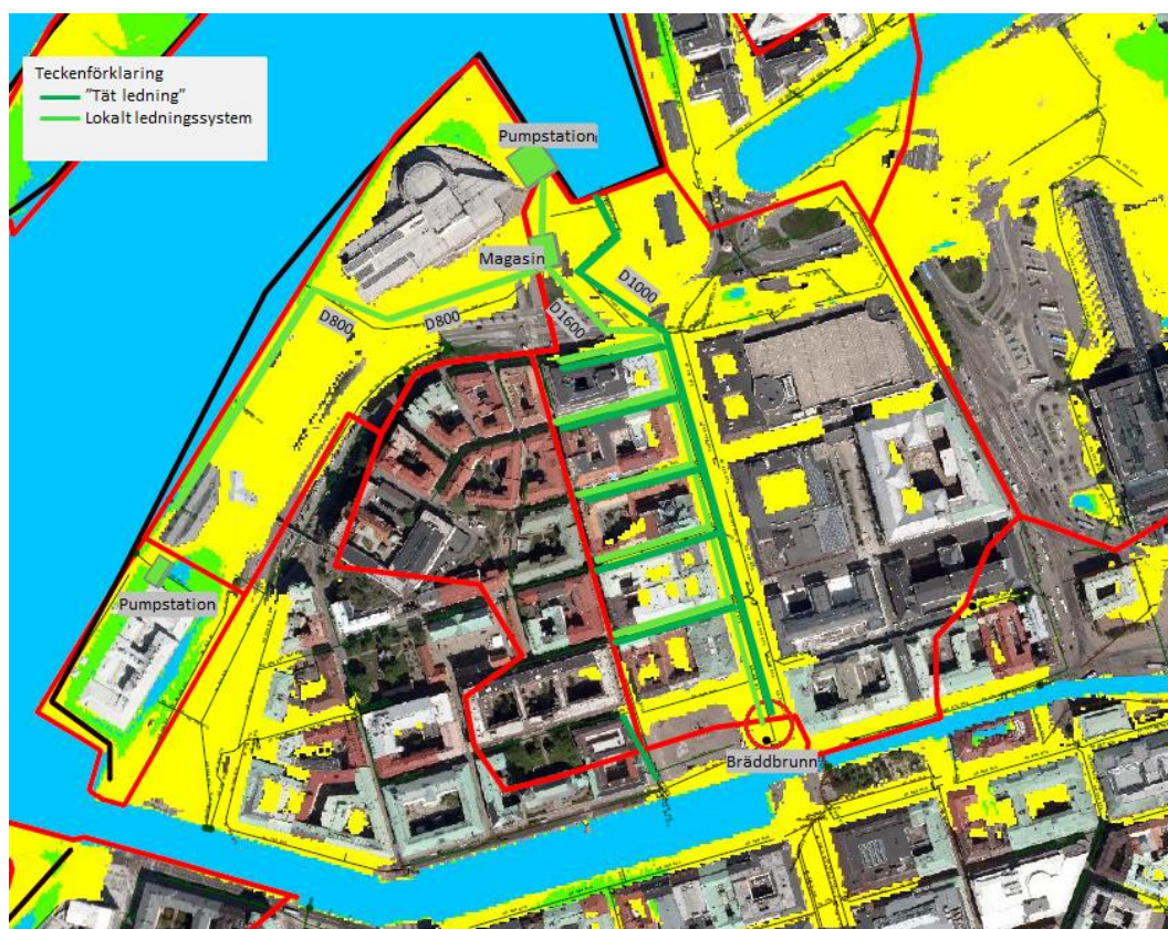
Figur 15. Förslag på ledningsutbyggnad och ledningsdimension för "täta ledningar" samt avskärande och lokala ledningar.
