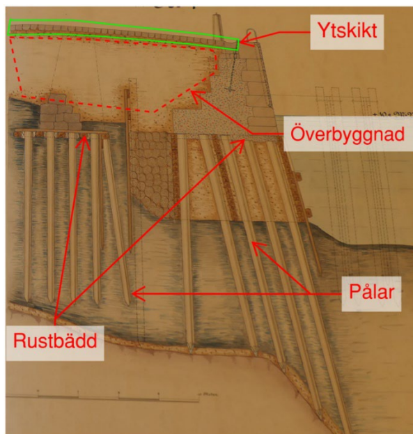
Principskiss kanalmur med definitioner, ur Kulturmiljöutredning Antiquum, 2021-11-22
