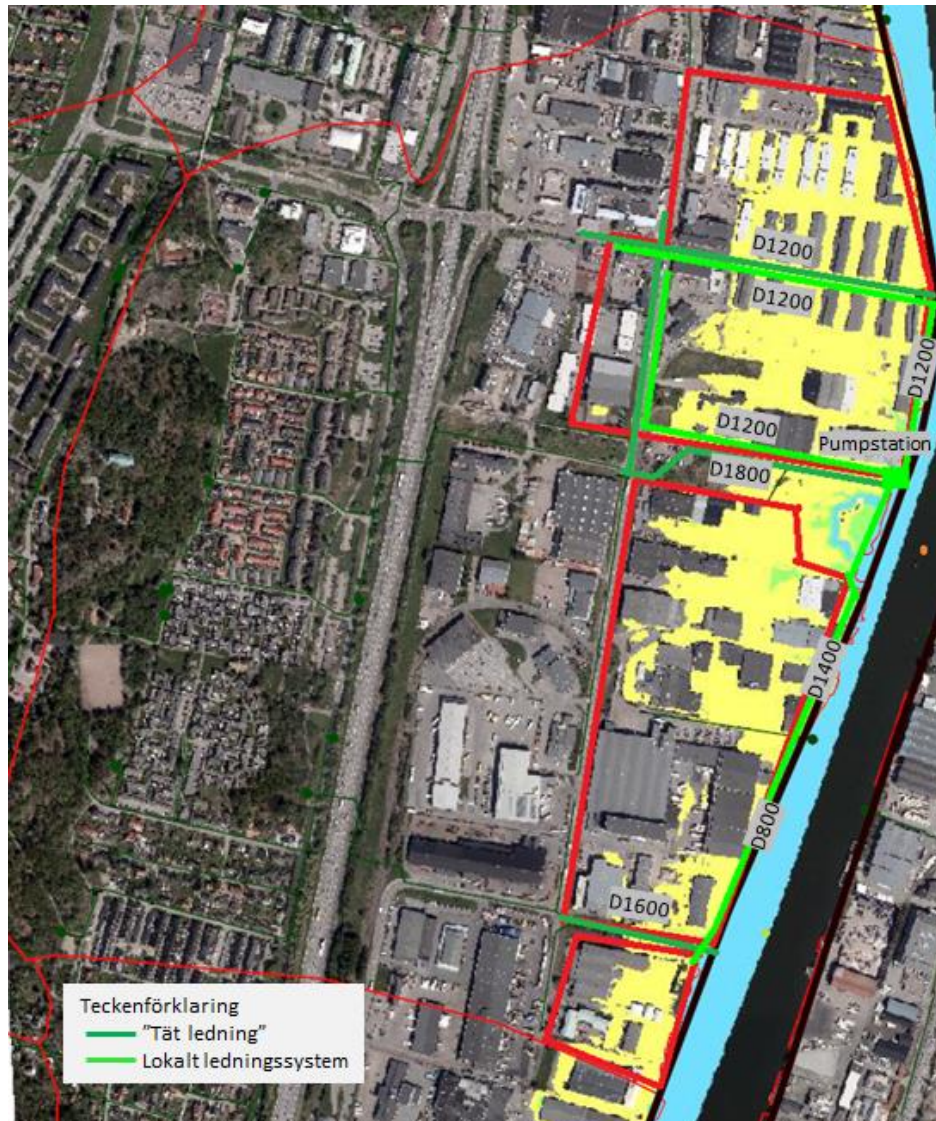
Figur 13. Förslag på ledningsutbyggnad och ledningsdimension för "täta ledningar" samt avskärande och lokala ledningar.
