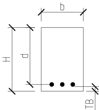
Figur 1 Principsnitt av en armerad betongkonstruktion
