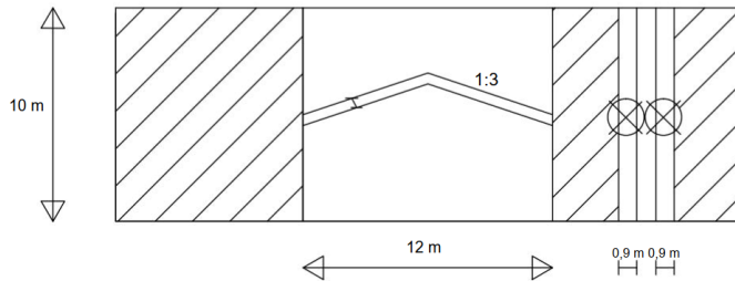
Figur 4. Principiell utformning av traditionell skydds/slussport, med slussport t.h.
