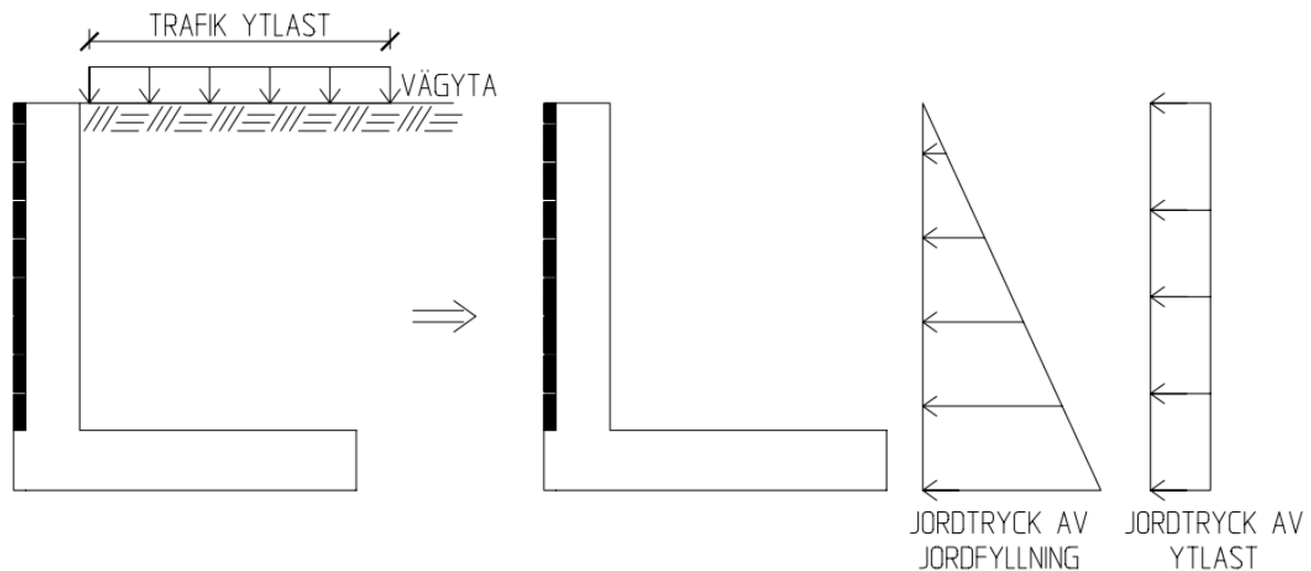
Figur 2 Stödmurkonstruktion utsatt för trafiklast
