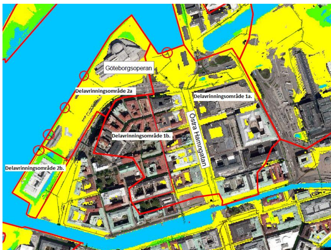
Figur 14. Delavrinningsområden samt fem utlopp (inringat i rött) inom Nordstans och Packhuskajens avrinningsområde.
