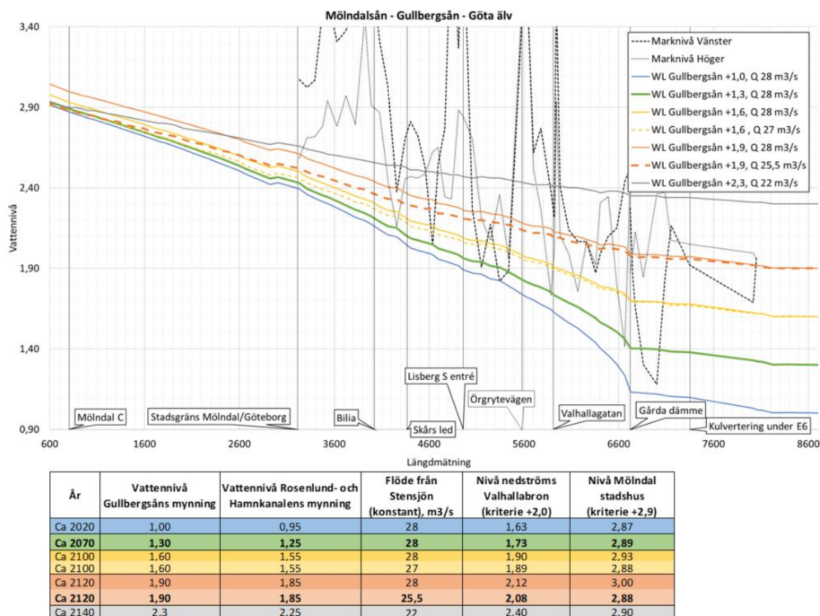
Figur 3-1. Vattenståndsprofiler från Mölndal C till Gullbergsåns mynning vid olika vattenstånd i havet och olika flöden
