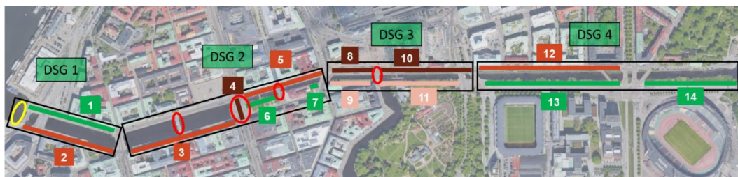
Programmets föreslagna indelning i fyra delsträcksgrupper visualiseras genom de svarta ramarna. Färgerna på delsträckorna inom respektive delsträcksgrupp anger graden av påverkan på kollektivtrafiken, ju mörkare desto större påverkan. Gul cirkel avser skydds-/slussportar för högvattenskydd.
