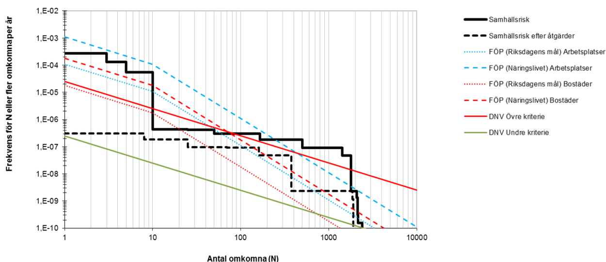
Figur 11. Uppskattad samhällsriskenivå utan (heldragen svart linje) och efter vidtagna åtgärder (streckad svart linje).
