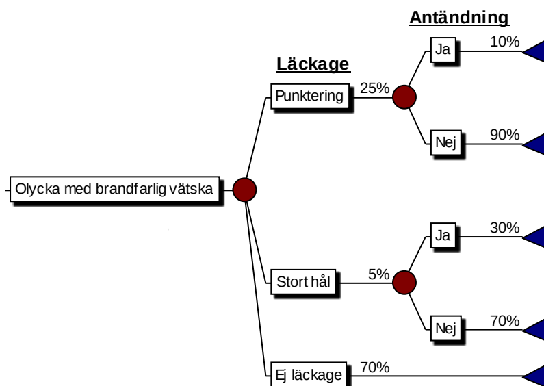
Figur 17. Händelseträd för farligt gods-olycka med brandfarlig vätska i lasten.
