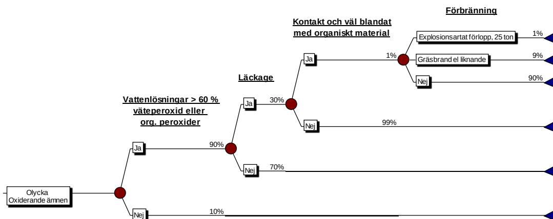
Figur 18. Händelseträd för farligt gods-olycka med oxiderande ämnen och organiska peroxider i lasten.
