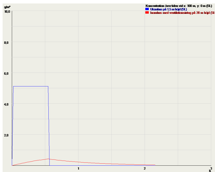
Figur 25. Koncentration utomhus och inomhus i förhållande till tiden efter olycka med \text{NH}_4 .
