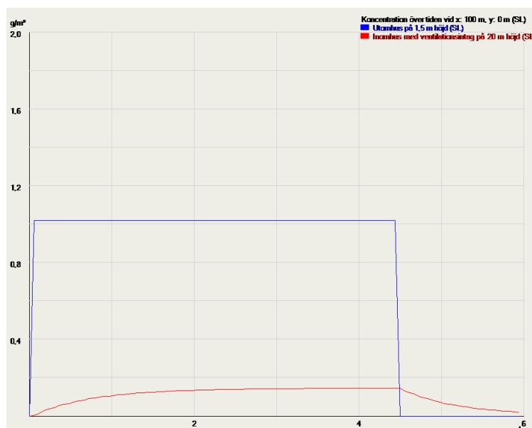
Figur 20. Koncentration utomhus och inomhus i förhållande till tiden efter olycka med SO 2 .
