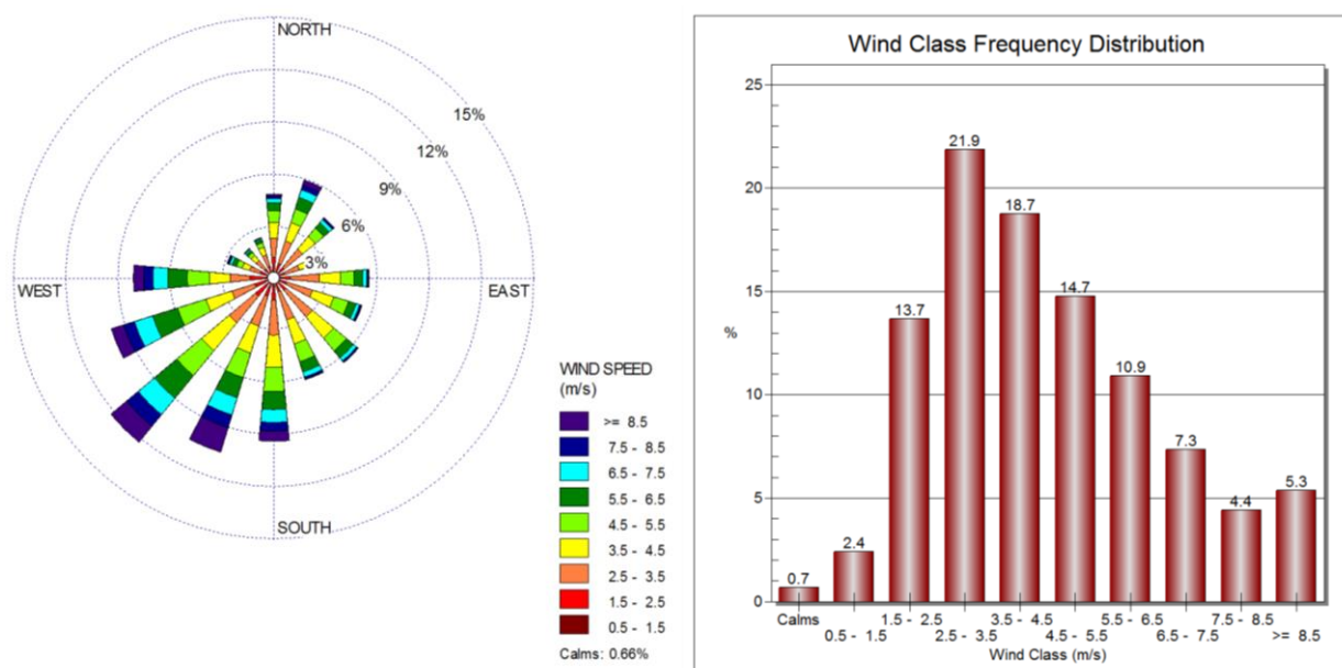
Figur 16. Vindros och vindhastighetsfördelning Landvetter flygplats 2003-2012. Medelvindhastighet 4.36 m/s [28].
