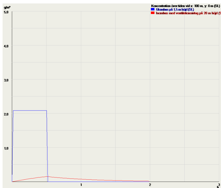
Figur 24. Koncentration utomhus och inomhus i förhållande till tiden efter olycka med Cl 2 efter 30 minuter, ventilationsintag är placerade 20 meter ovan mark.
