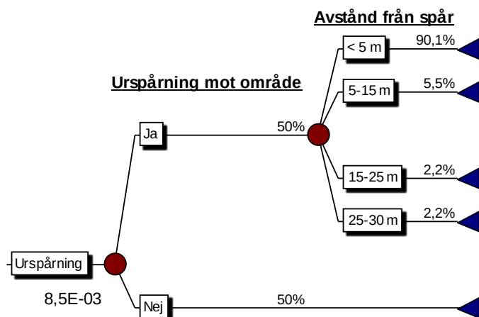
Figur 12. Händelseträd med sannolikheter för urspårningar.
