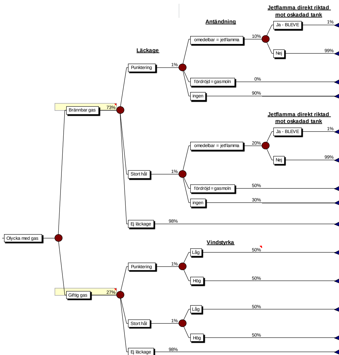
Figur 15. Händelseträd för farligt gods-olycka med gas i lasten.
